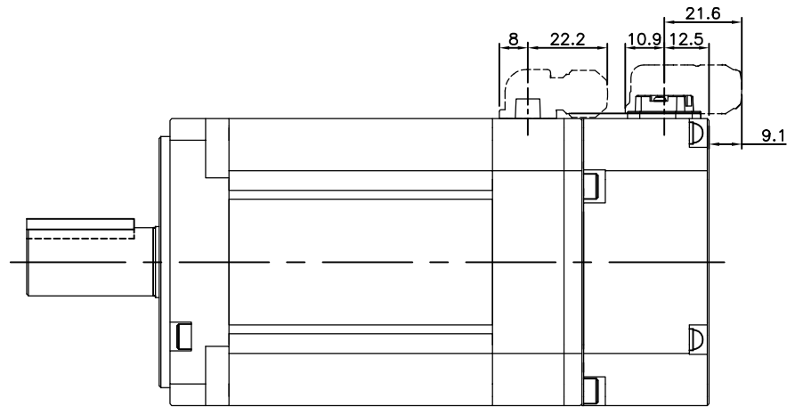
<Cable 인출 방향이, 축 반대 방향일 경우>
