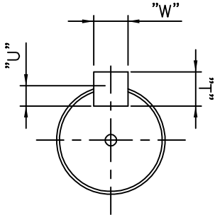
<축단 상세도, S/C 2:1>
