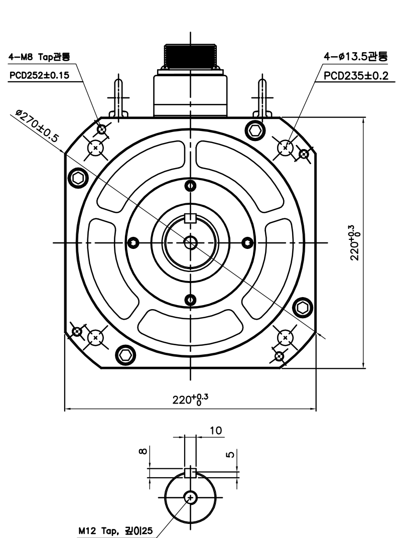
<축단 치수 상세도>
