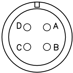
<시양:MS3102A32-17P>
