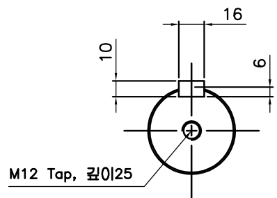
<축단 치수 상세도>
