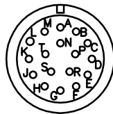
<사양:MS3102A20-29P>
